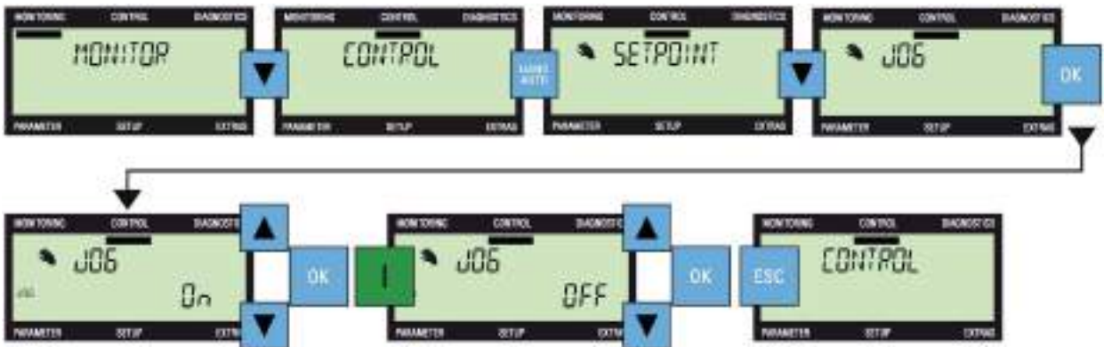
Figura 7-3 Función Jog
